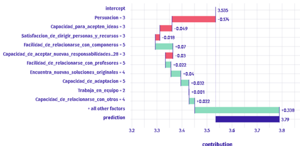
Figura 7. Modelo predictivo
